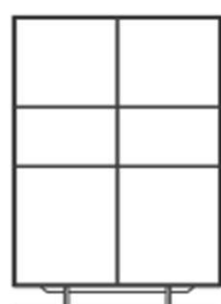
NYR VIT HOOG NR. 408 B 1128 mm / H 1747 mm / D 475 mm
