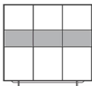
NYR VIT HOOG NR. 413 B 1682 mm / H 1747 mm / D 475 mm
