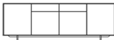
NYR DRES NR. 232 B 2236 mm / H 862 mm / D 475 mm
