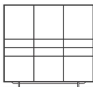
NYR VIT HOOG NR. 417 B 1682 mm / H 1747 mm / D 475 mm
