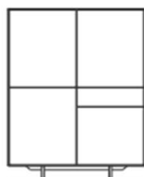
NYR VIT LAAG NR. 313 B 1128 mm / H 1570 mm / D 475 mm
