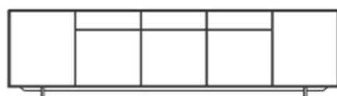
NYR DRES NR. 248 B 2790 mm / H 862 mm / D 475 mm
