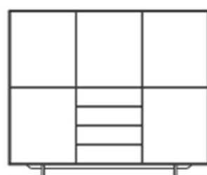
NYR VIT LAAG NR. 317 B 1682 mm / H 1570 mm / D 475 mm
