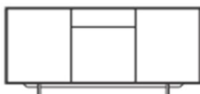
NYR DRES NR. 227 B 1682 mm / H 862 mm / D 475 mm
