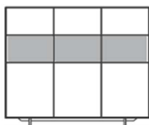
NYR VIT LAAG NR. 319 B 1682 mm / H 1570 mm / D 475 mm
