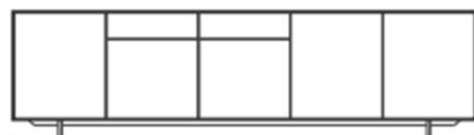
NYR DRES NR. 243 B 2790 mm / H 862 mm / D 475 mm
